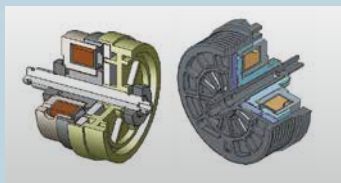
実機断面図
