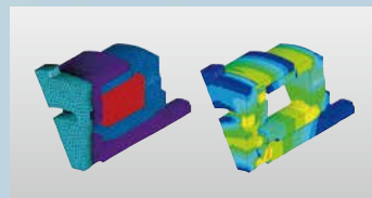
FEM解析実施例
